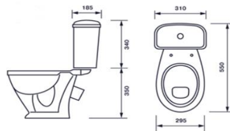
Рисунок 1. Чертеж унитаза
