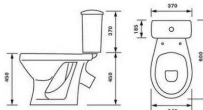
Рисунок 1. Чертеж унитаза
