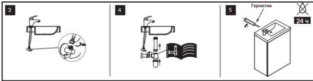
Рисунок 3. Установка раковины. Крепление на тумбу
