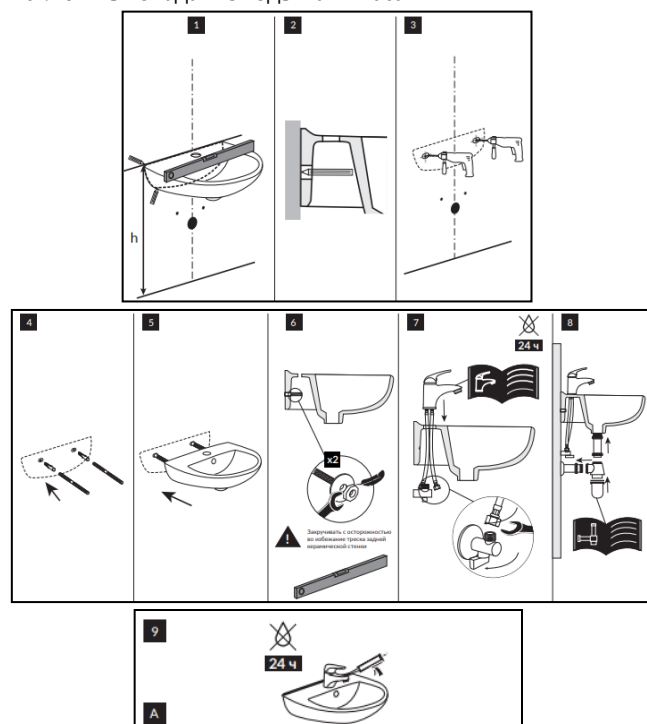
Рисунок 2. Установка раковины. Крепление к стене
