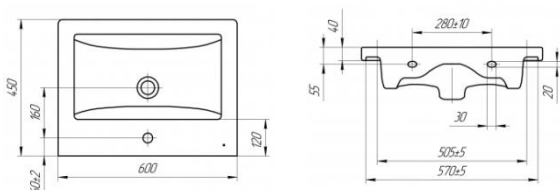
Рисунок 1. Чертеж раковины
