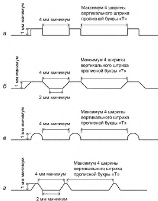
Рисунок 4 — Параметры шрифтовых знаков и рельефа (рифа) РЛШ
