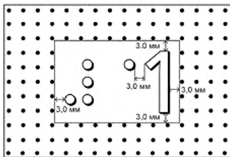
Рисунок 42 — Свободное пространство вокруг меток, встроенных в текстуру
