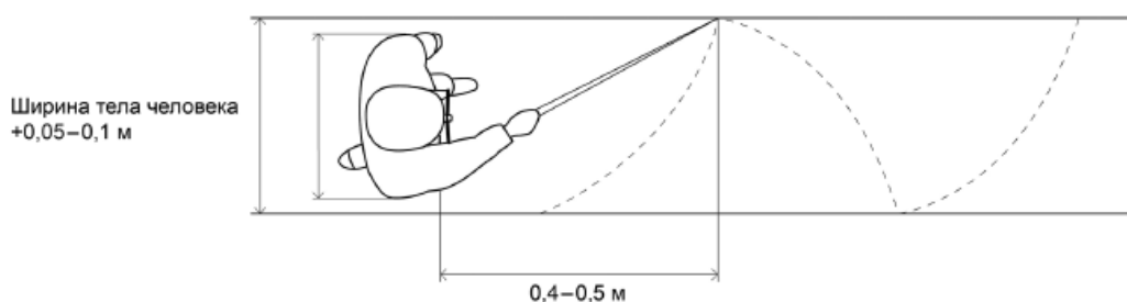
Рисунок В.1 - Зона действия белой трости
