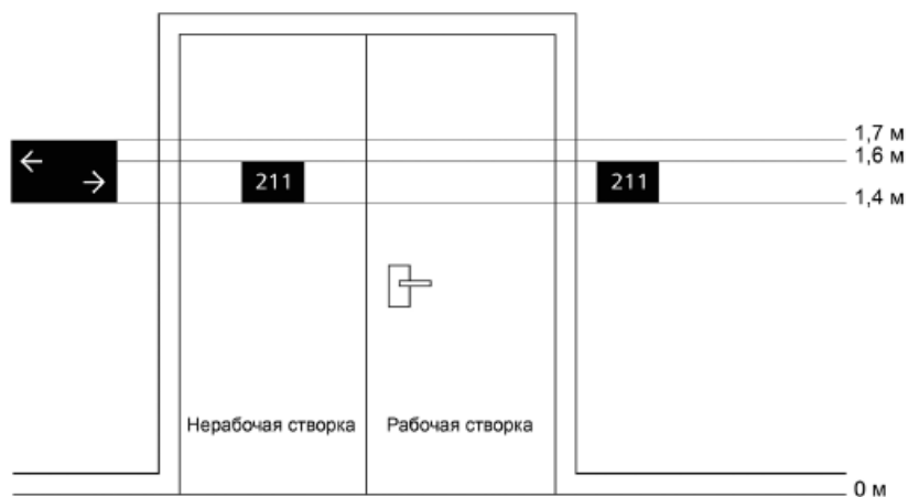
Рисунок 8 - Вариант размещения информации на нерабочих створках дверей
