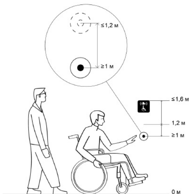
Рисунок 36 - Высота размещения кнопки вызова и информирующей таблички
