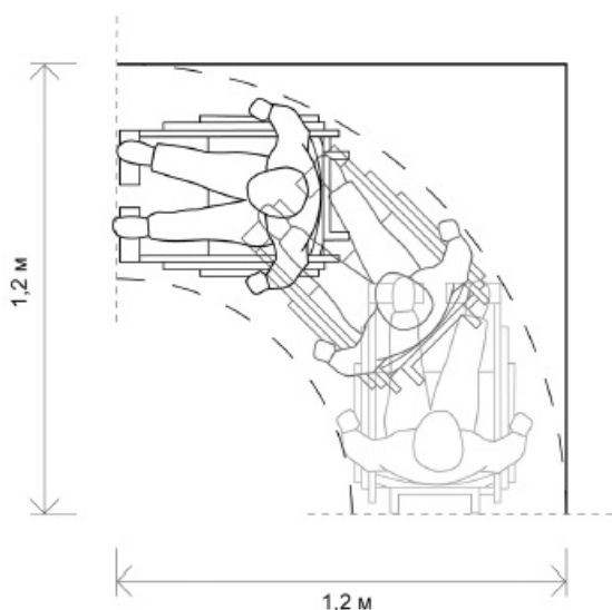
Рисунок Б.2 - Пространство для поворота на 90°
