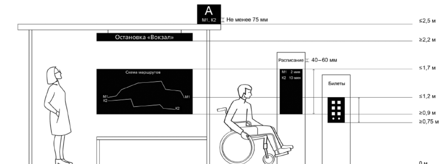
Рисунок 29 - Параметры размещения средств информации на остановочных пунктах
