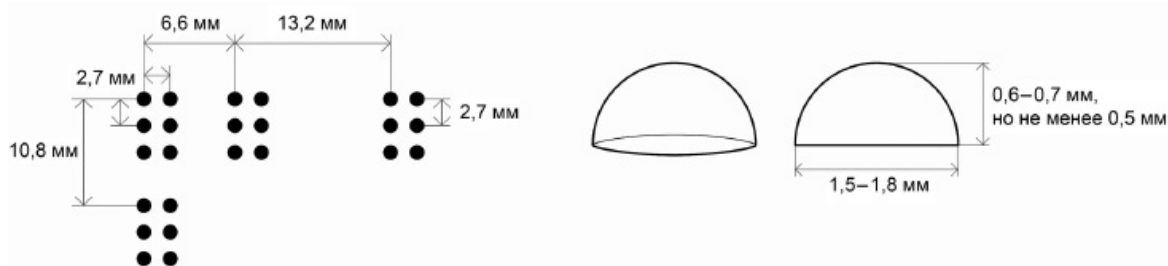
Рисунок 31 - Размеры рельефно-точечного шрифта Брайля
