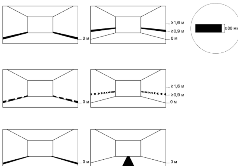
Рисунок 27 - Визуальная направляющая разметка
