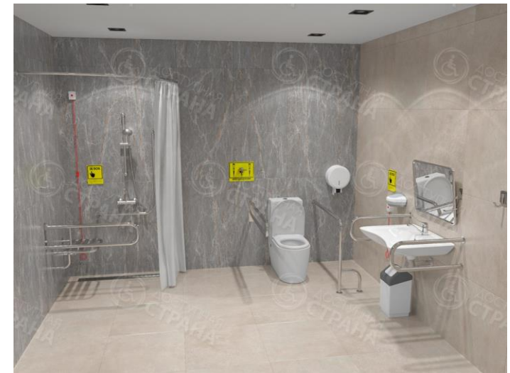
Комплект оборудования для санузла и душевой для инвалидов по ГОСТ (центральное расположение унитаза, унитаз арт. 4620)
