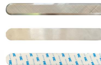
Тактильный индикатор из нержавеющей стали полоса 35мм 280x35x5мм на самоклеящейся основе, арт. 2645
