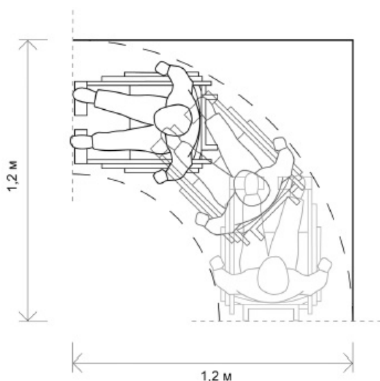
Рисунок Б.2 - Пространство для поворота на 90^\circ
