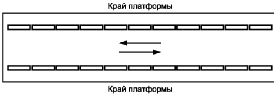
Рисунок А.4 — Форма рифления — одноэлементная тактильная полоса с плоской вершиной (шумлиния), используемая для обустройства протяженных предупреждающих ТНУ вдоль края платформ различного назначения
