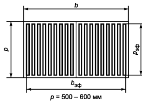
Рисунок А. 1 — Форма рифления — прямолнейные параллельные рифы с плоской вершиной , используемые для обустройства предупреждающих ТНУ перед выходом с тротуара на пешеходные переходы и при пересечении местных проездов
