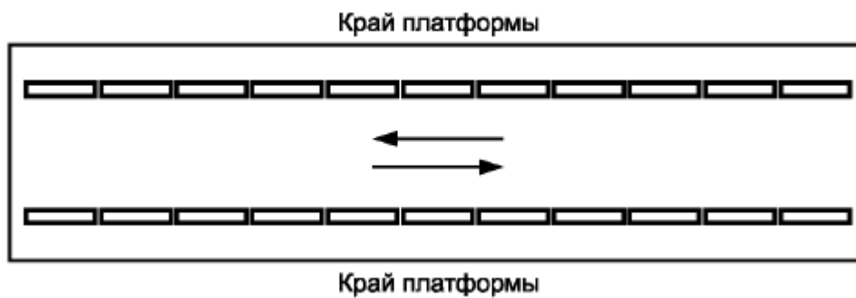
Рисунок А.4 — Форма рифления — одноэлементная тактильная полоса с плоской вершиной (шущлиния), используемая для обустройства протяженных предупреждающих ТНУ вдоль края платформ различного назначения
